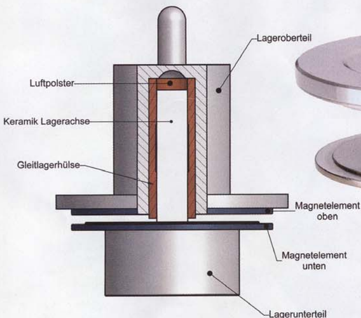
Der Plattenteller schwebt fast völlig reibungsfrei auf Clearaudios neuem Magnetlager und ist so wirksam entkoppelt. Der Unterschied zu anderen magnetischen Lagern besteht vor allem in der Lagerachse aus Keramik
