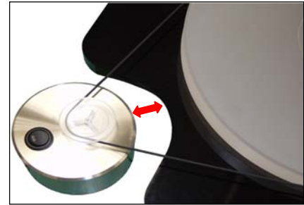
Abbildung 5: Ausrichten des Motors
