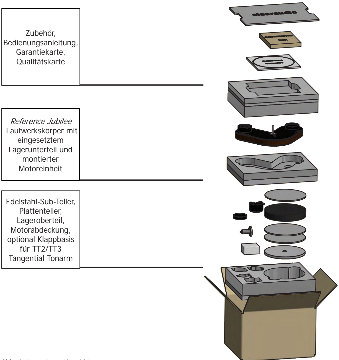
Abb. 1: Verpackungsübersicht
