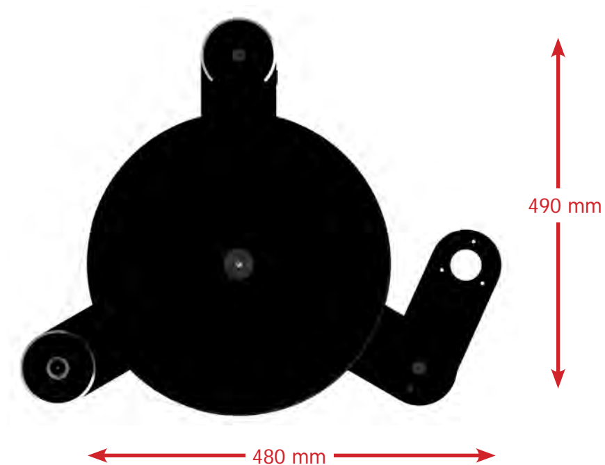
Abb. 3: Aufstellfläche Innovation Basic
