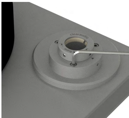
Abb. 3a: Montage der swing base
