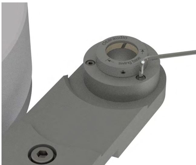
Abb. 5a: Montage der swing base
