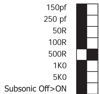
Abb. 2.3: Einstellung Ziel 500 Ohm
