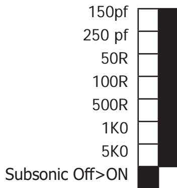
Abb. 2.2: Grundeinstellung
