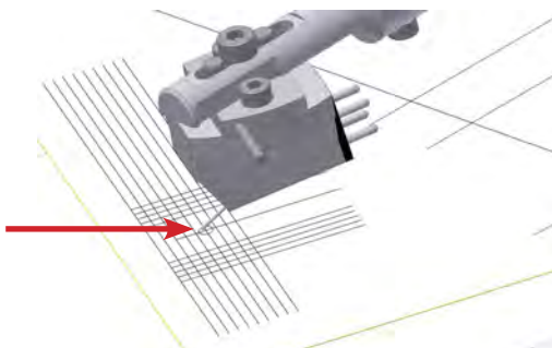
Abb. 11: Korrekte Position des Abtastdiamanten
