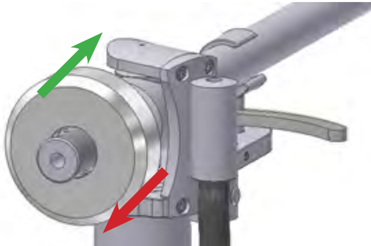
Abb. 12: Einstellung der Auflagekraft
