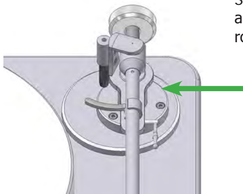
Abb. 7: Einstellung der Tonarmhöhe
