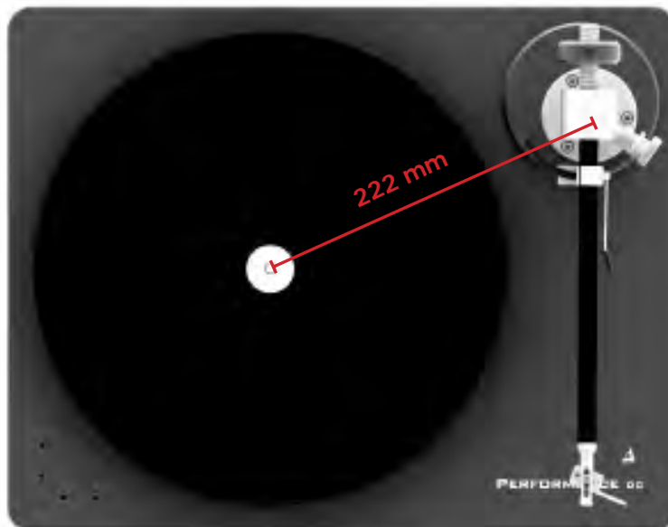
Abb. 6: Abstand der Spindel zum Drehpunkt des Tonarms
